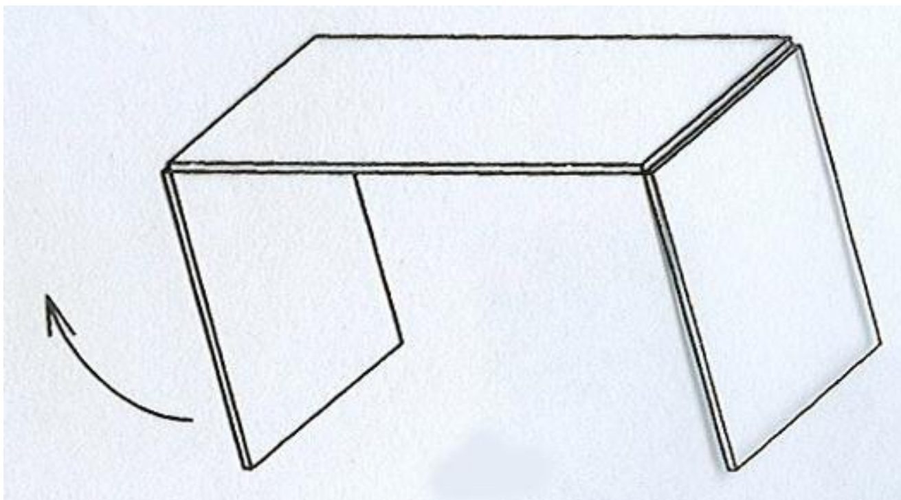
Zavesená prídavná st. doska
